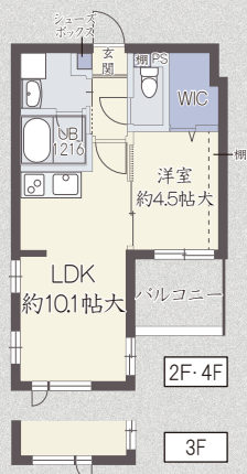
A1 type 1LDK ■専有面積 37.58㎡ ■バルコニー面積 4.70㎡
