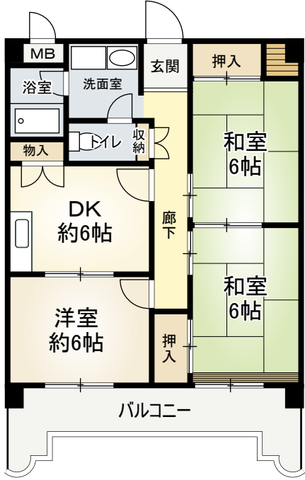
Aタイプ 3DK 60.48㎡
