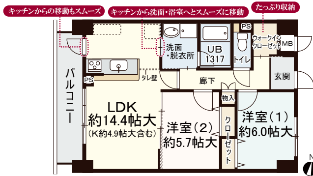
B3 type/2LDK/ 専有面積 63.31㎡ バルコニー面積 7.95㎡
