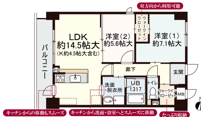
C2 type/2LDK/ 専有面積 63.31㎡ バルコニー面積 8.47㎡
