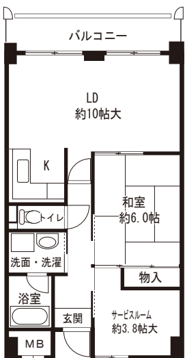
C type | 1LDK+S ※1 ■専有面積 51.19㎡
